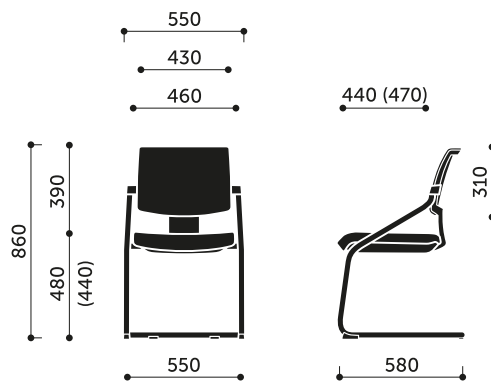
20V / 20VN
