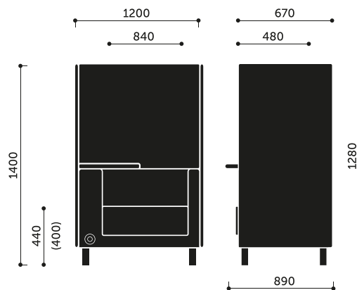
VL1,5 HW / VL1,5 VW + VL W1
