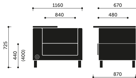
VL1,5 H / VL1,5 V
